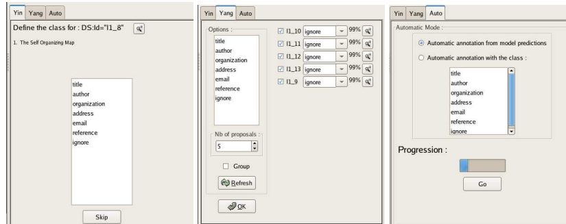
Figure 5. Les 3 panneaux d'annotation de l'interface.
