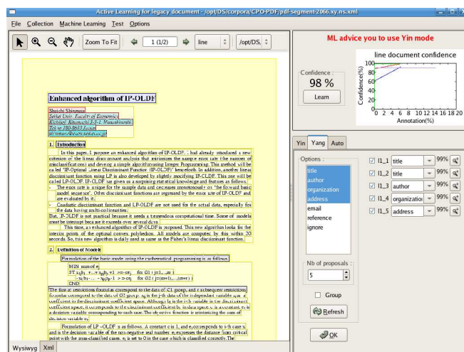
Figure 4. Vue d’ensemble de ALDAI.
