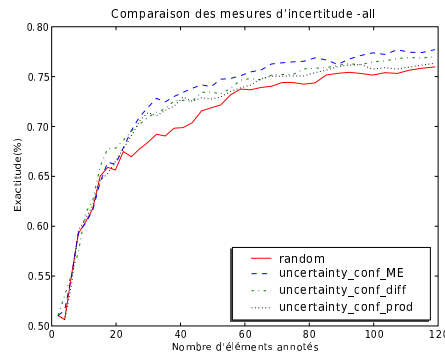
Figure 3. Moyenne des évaluations sur 10 documents d'UCI.
