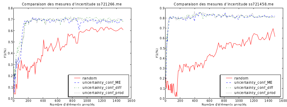
Figure 2. Evaluation sur une série de documents techniques
