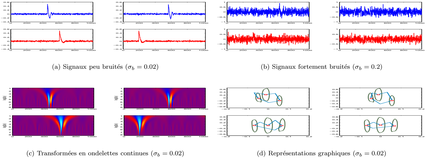
FIG. 1 – Les 4 représentations graphiques du haut sont de la classe 1 ( u = 1 \cdot 10^{-3}, v = 2 \cdot 10^{-3} ), les 4 du bas sont de la classe -1. ( u = 5 \cdot 10^{-4}, v = 6 \cdot 10^{-4} )
